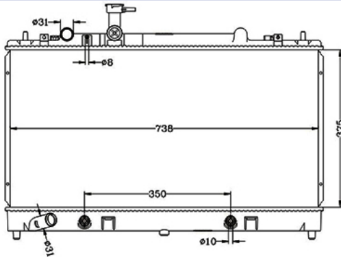
COD: 14182 RADIADOR MAZDA 6 M/NUEVO AUTOMATICO LAMINILLA
