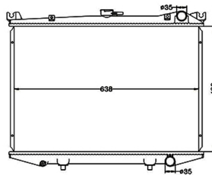
COD: 14546 RADIADOR NISSAN D21 96/ MECANICA LAMINILLA
