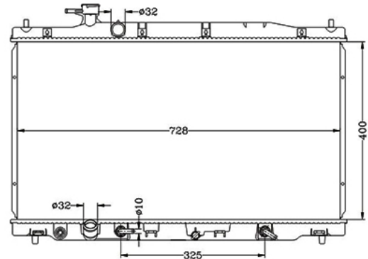
COD: 14535 RADIADOR HONDA CRV 2.4 PILOT 07-08 AUTOMATICO LAMINILLA
