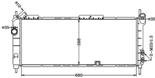
COD: 6292 RADIADOR CHEVROLET CORSA 95 GASOLINA LAMINILLA
