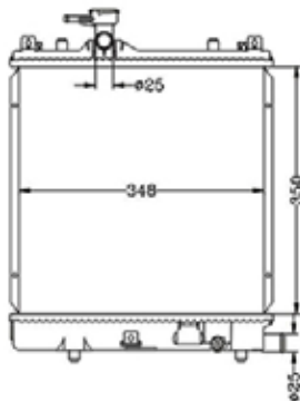
COD: 13599 RADIADOR CHEVROLET ALTO LAMINILLA
