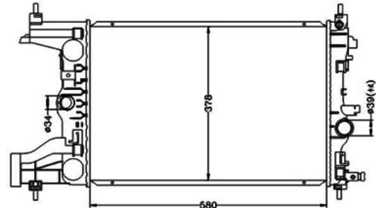
COD: 9698 RADIADOR CHEVROLET CRUZE 1.8 MECANICO
