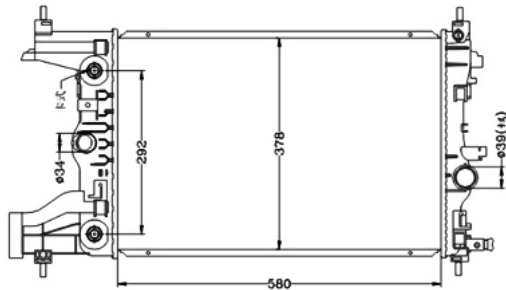
COD: 9982 RADIADOR CHEVROLET CRUZE 1.8 AUTOMATICO
