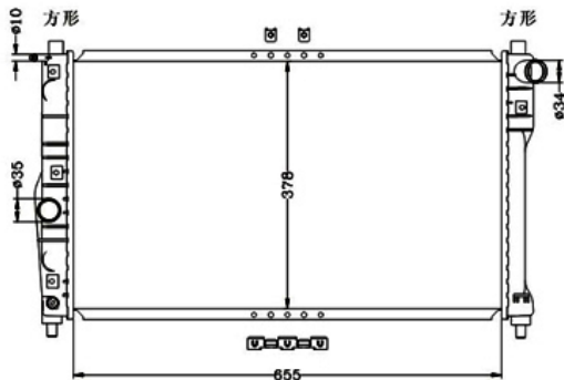
COD: 8437 RADIADOR DAEWOO NUBIRA 98/ LAMINILLA
