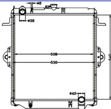
COD: 13609 RADIADOR TOYOTA MACHO 4.5 LAMINILLA
