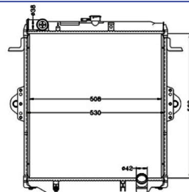
COD: 13610 RADIADOR TOYOTA MACHO DIESEL 4.5 LAMINILLA
