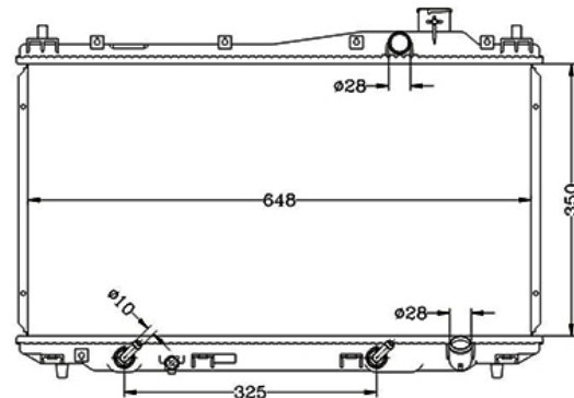
COD: 14533 RADIADOR HONDA CIVIC 01-05 AUTOMATICO LAMINILLA
