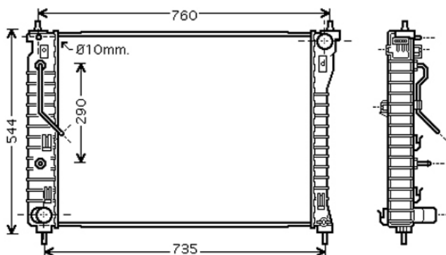
COD: 13732 RADIADOR CHEVROLET CAPTIVA 2.4 3.2 A/A AUTOMATICO LAMINILLA
