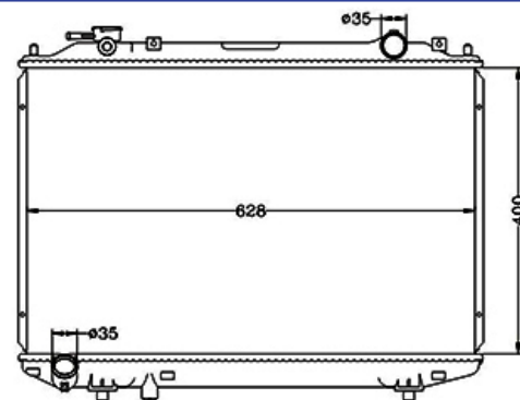
COD: 12502 RADIADOR MAZDA B2200 INYECCION LAMINILLA
