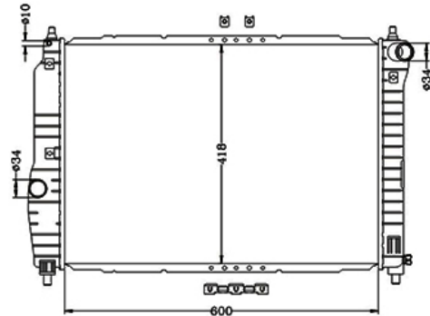
COD: 3458 RADIADOR CHEVROLET AVEO CON A/A LAMINILLA
