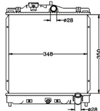
COD: 14023 RADIADOR HONDA CIVIC 92-00 MECANICO LAMINILLA
