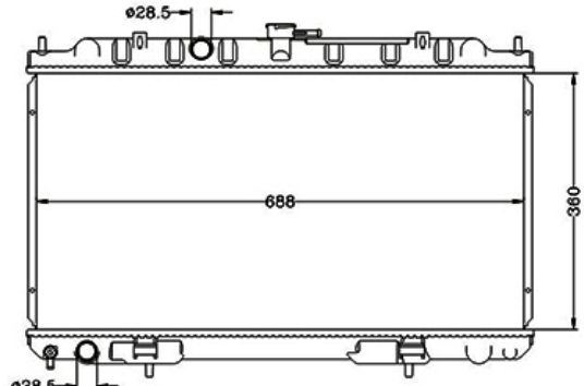
COD: 14028 RADIADOR NISSAN ALMERA MECANICO LAMINILLA
