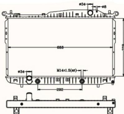
COD: 14017 RADIADOR CHEVROLET EPICA 2.5 AUTOMATICO LAMINILLA
