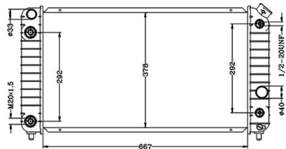
COD: 12500 RADIADOR CHEVROLET BLAZER 96
