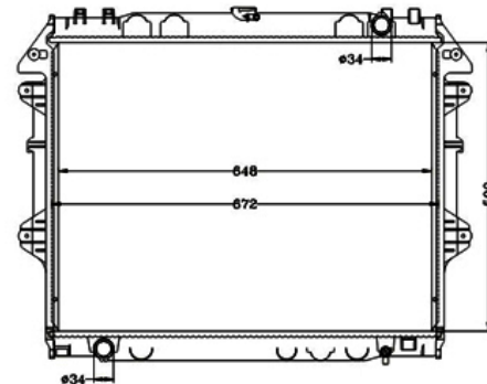
COD: 12821 RADIADOR TOYOTA HILUX 2.7 GASOLINA LAMINILLA
