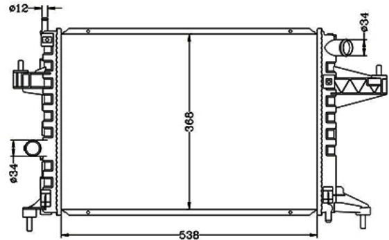
COD: 10354 RADIADOR CHEVROLET CORSA EVOLUTION 1.4 LAMINILLA
