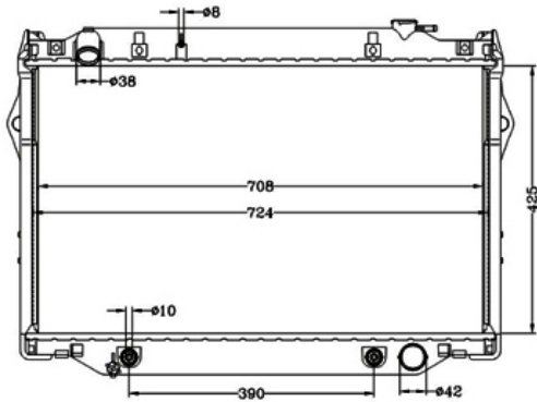
COD: 13607 RADIADOR TOYOTA BURBUJA AUTOMATICA LAMINILLA
