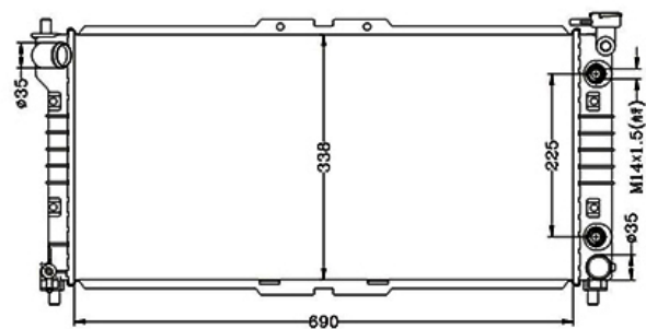
COD: 11034 RADIADOR MAZDA 626 MILENIUM AUTOMATICO LAMINILLA
