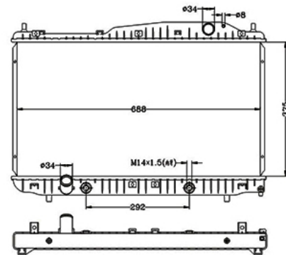
COD: 14018 RADIADOR CHEVROLET EPICA AUTOMATICO LAMINILLA
