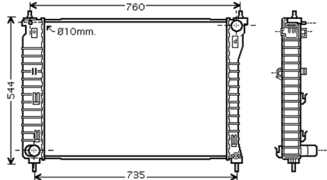
COD: 13733 RADIADOR CHEVROLET CAPTIVA 2.4 3.2 A/A AUTOMATICO LAMINILLA
