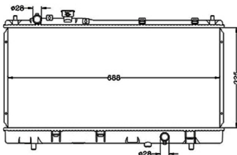
COD: 10785 RADIADOR MAZDA ALLEGRO 1.3/1.6 LAMINILLA
