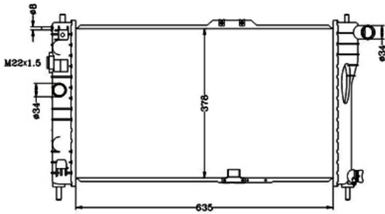
COD: 3117 RADIADOR DAEWOO CIELO TANQUE GRUESO LAMINILLA
