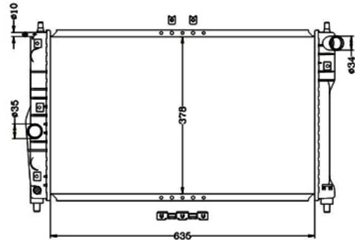
COD: 6280 RADIADOR DAEWOO LANOS CON A/C LAMINILLA 63.5 cm
