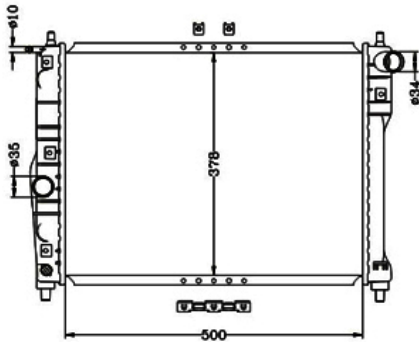
COD: 668 RADIADOR DAEWOO LANOS SIN A/A LAMINILLA 50 cm
