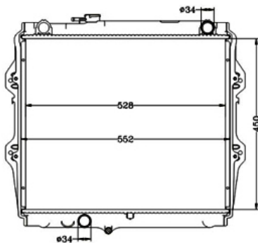
COD: 13608 RADIADOR TOYOTA HILUX RAIDER LAMINILLA
