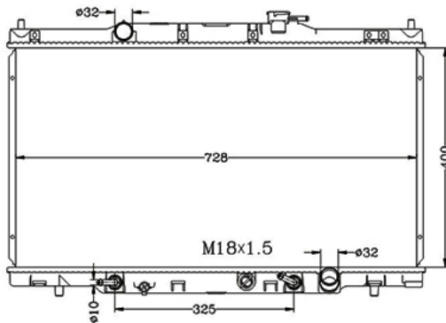
COD: 14534 RADIADOR HONDA CRV 02-06 AUTOMATICO LAMINILLA
