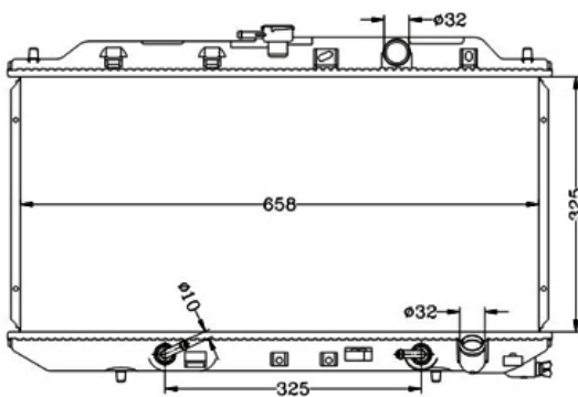
COD: 14178 RADIADOR HONDA INTEGRA 90-93 AUTOMATICO LAMINILLA
