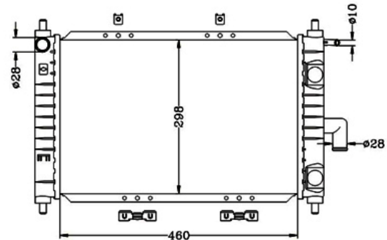
COD: 10029 RADIADOR DAEWOO MATIZ SPARK 7/24 QQ LAMINILLA
