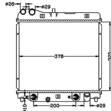
COD: 14536 RADIADOR HONDA FIT AUTOMATICO LAMINILLA
