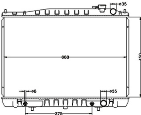
COD: 13605 RADIADOR NISSAN FRONTIER AUTOMATICA GASOLINA DIESEL LAMINILLA
