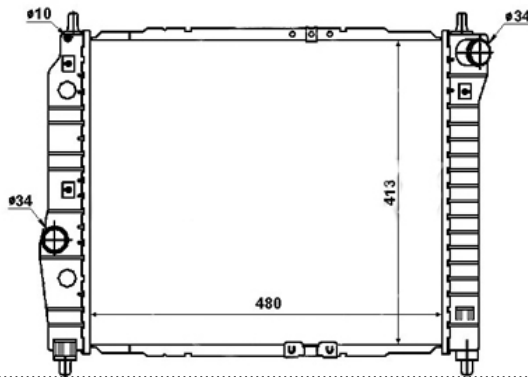
COD: 11274 RADIADOR CHEVROLET AVEO S/AIRE PMC
