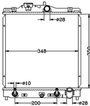
COD: 14022 RADIADOR HONDA CIVIC 92-00 AUTOMATICO LAMINILLA
