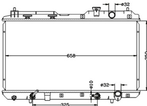
COD: 14024 RADIADOR HONDA CRV 97-01 AUTOMATICO LAMINILLA
