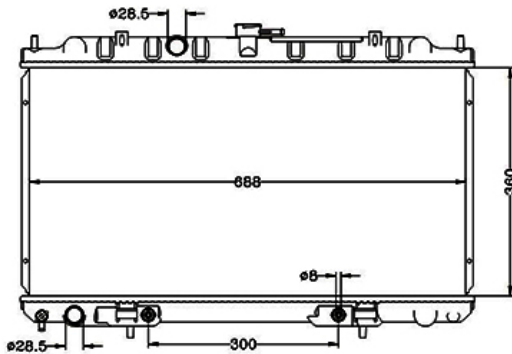
COD: 14078 RADIADOR NISSAN ALMERA AUTOMATICO LAMINILLA
