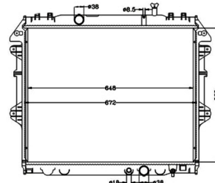
COD: 12820 RADIADOR TOYOTA HILUX VIGO LAMINILLA
